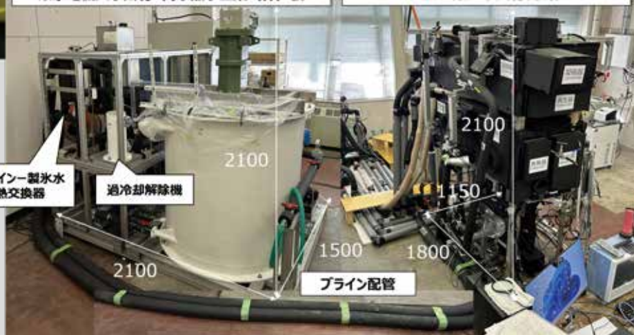
3kW氷点下冷熱用吸収冷凍機 八戸工業大学所有、製作
