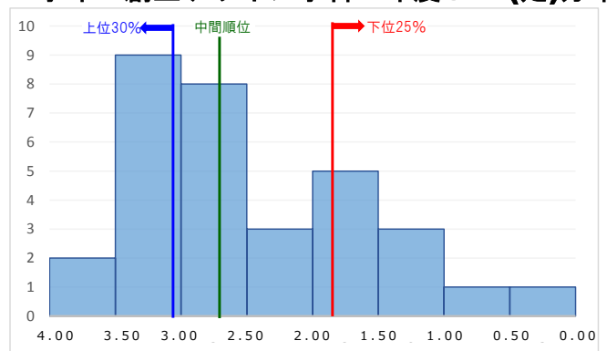
4学年 創生デザイン学科 年度GPA(定)分布
