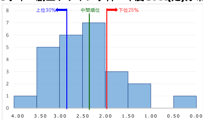
3学年 創生デザイン学科 年度GPA(定)分布
